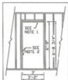
EXT. DOOR FRAMING DETAIL
